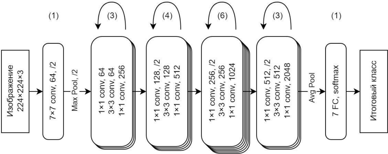
Архитектура ИНС ResNet50
