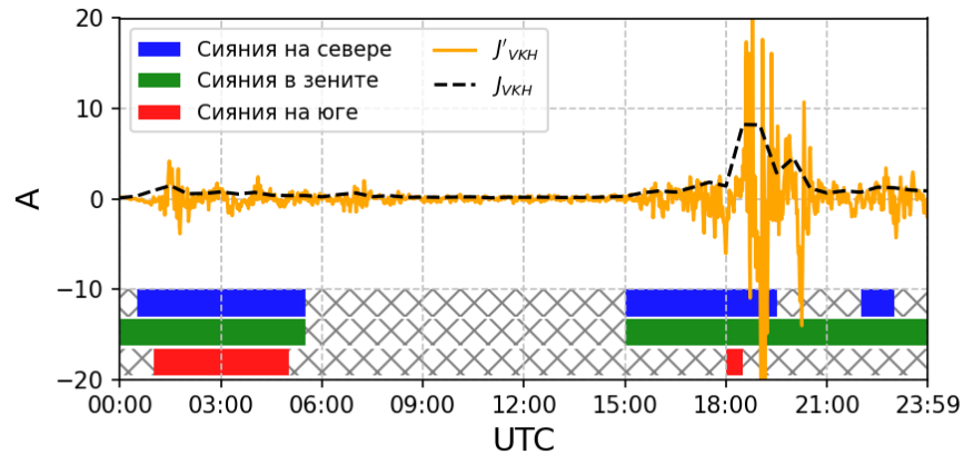
Сопоставление уровня ГИТ на станции VKN и области возникновения сияний в окрестности обсерватории LOZ (по состоянию на 14.12.2013 г.)
