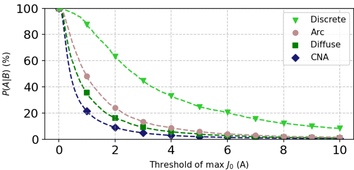
Вероятный уровень ГИТ относительно наблюдаемой структуры полярных сияний
