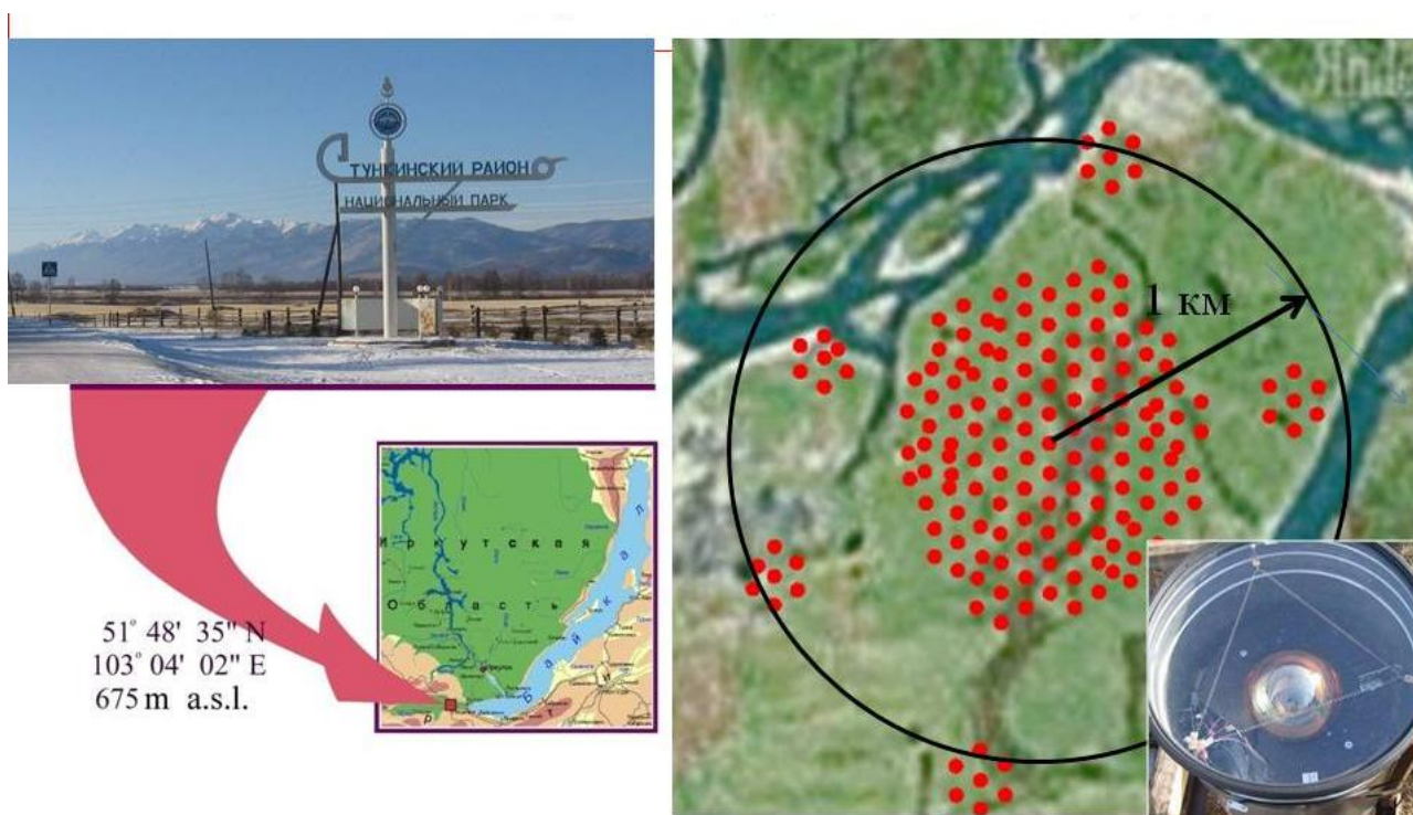
Рис.1 Установка Тунка-133
